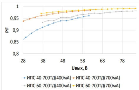
Зависимость коэффициента мощности от выходного напряжения
