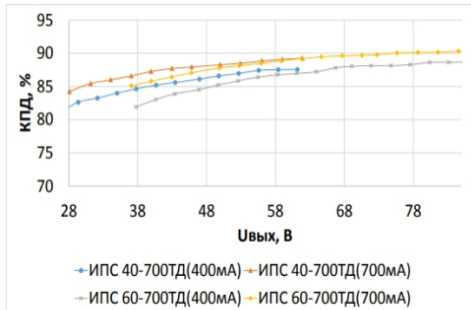
Зависимость КПД от выходного напряжения
